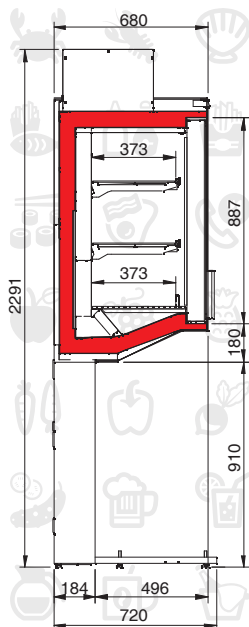
Sovrastruttura standard Standard top structure
