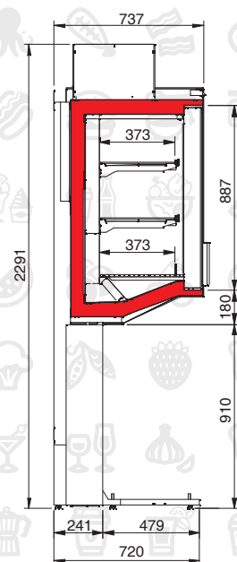
Sovrastruttura autoportante Self-bearing top structure
