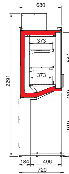
Sovrastuttura standard Standard top structure
