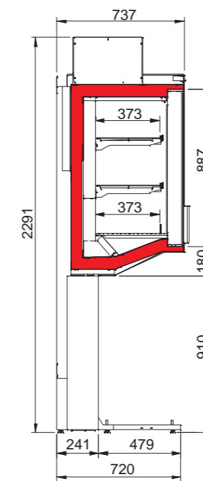
Sovrastuttura autoportante Self-bearing top structure
